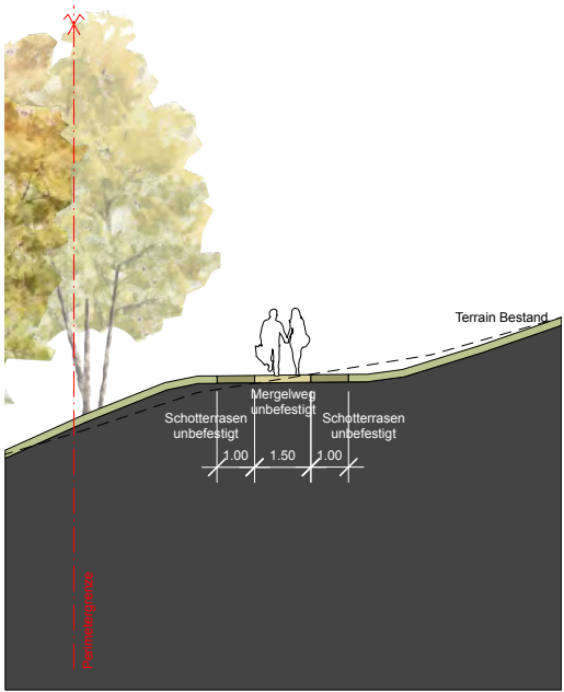
Schnitt B
