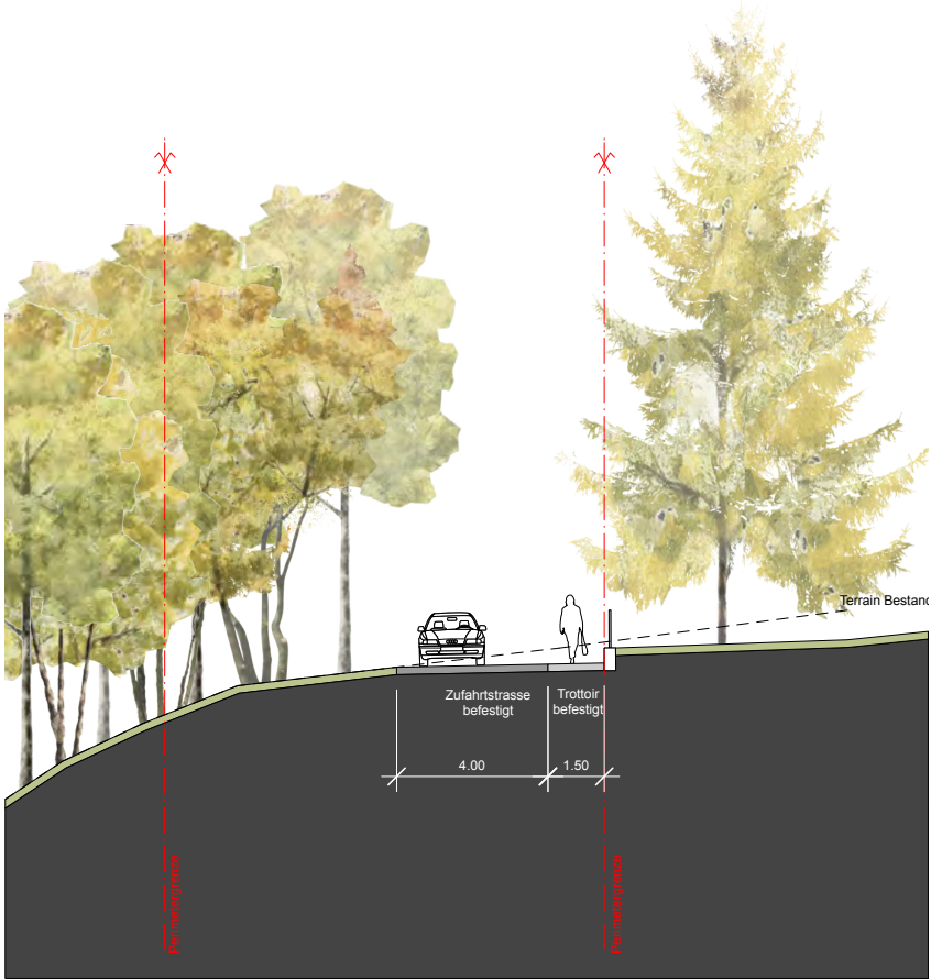
Schnitt A
